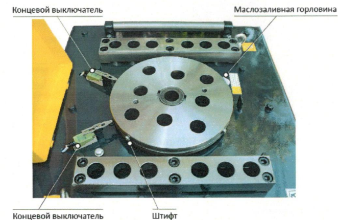
Рис. 3Б Вид с поднятой крышкой GW 40A
