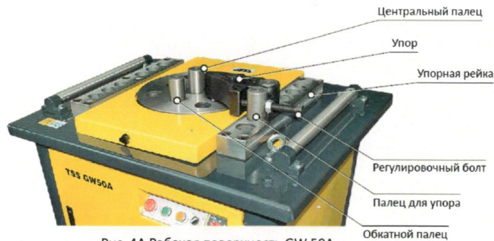
Рис. 4А Рабочая поверхность GW 50А
